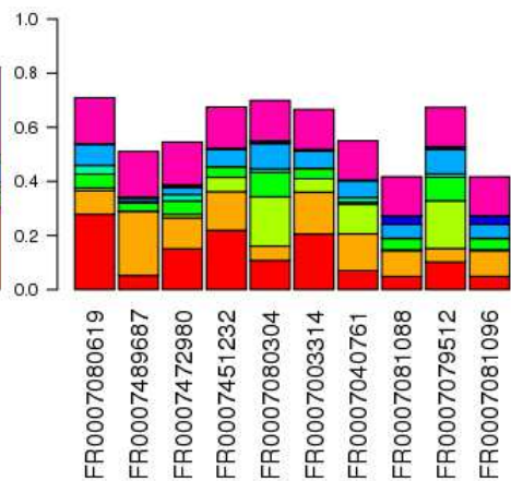
Valeurs_PCA 9
