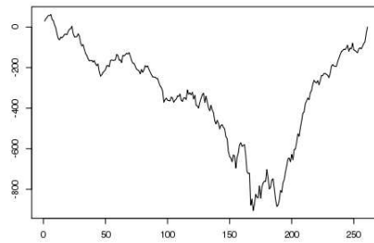
PCA_2
