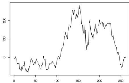
PCA_4
