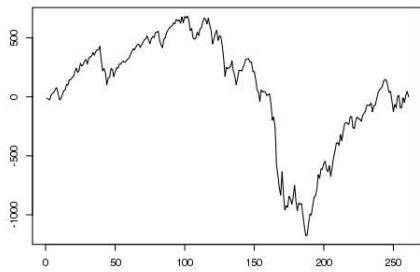
PCA_1
