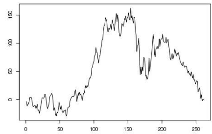
PCA_9
