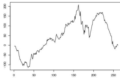
PCA_8
