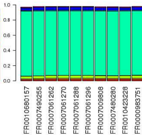
Valeurs_PCA 8
