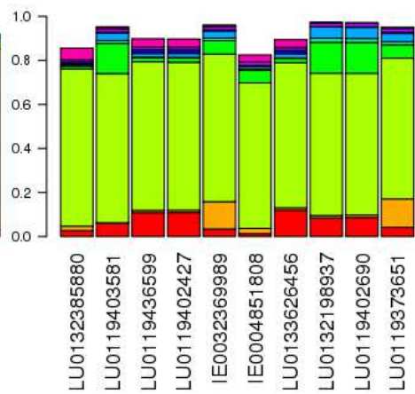
Valeurs_PCA 6
