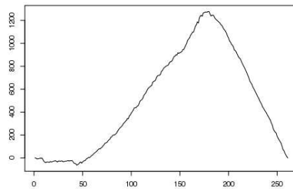
PCA_5
