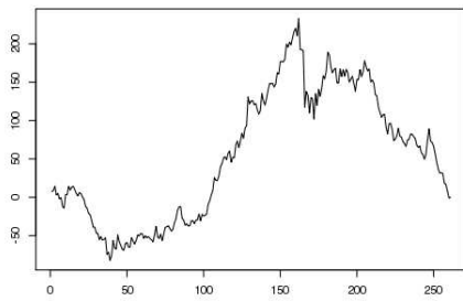
PCA_7
