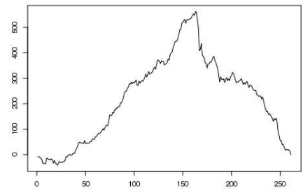
PCA_6
