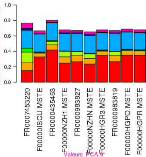
Valeurs_PCA 9
