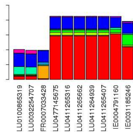
Valeurs_PCA 7
