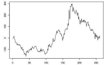
PCA_3
