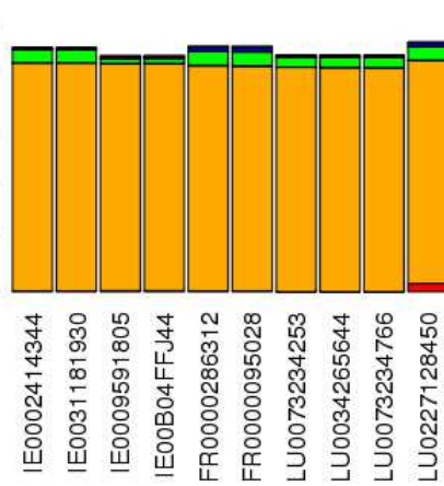
Valeurs_PCA 5
